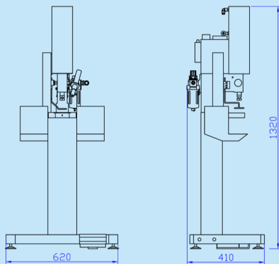
機身外形尺寸圖 Machine external dimensions diagram
